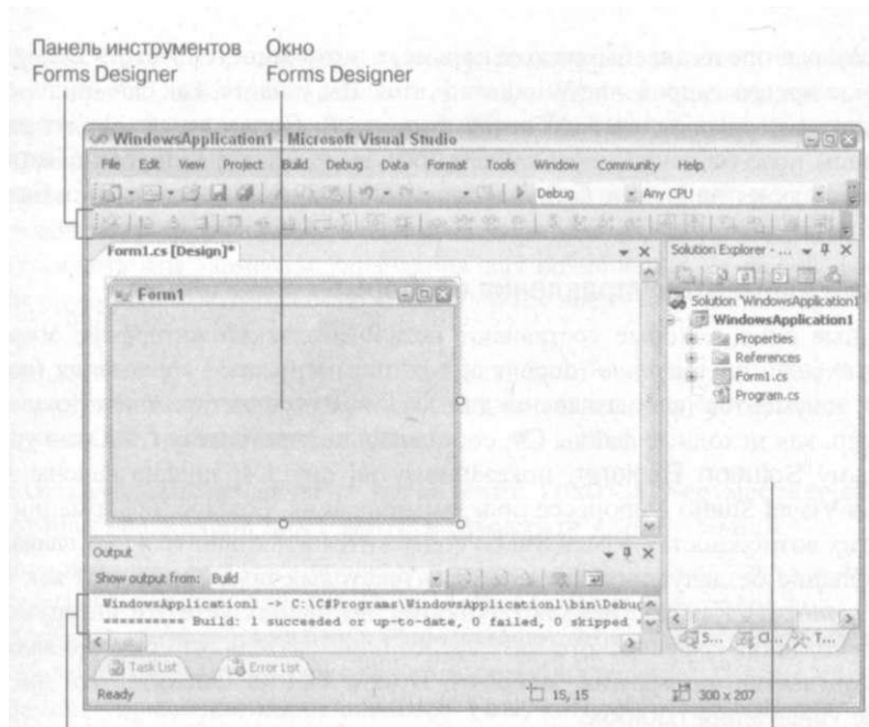
Окно вывода
