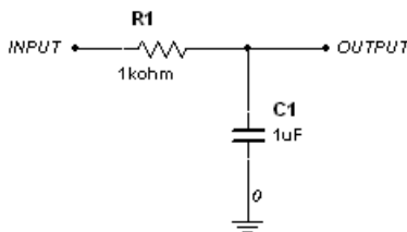
P1a (Circuit)
